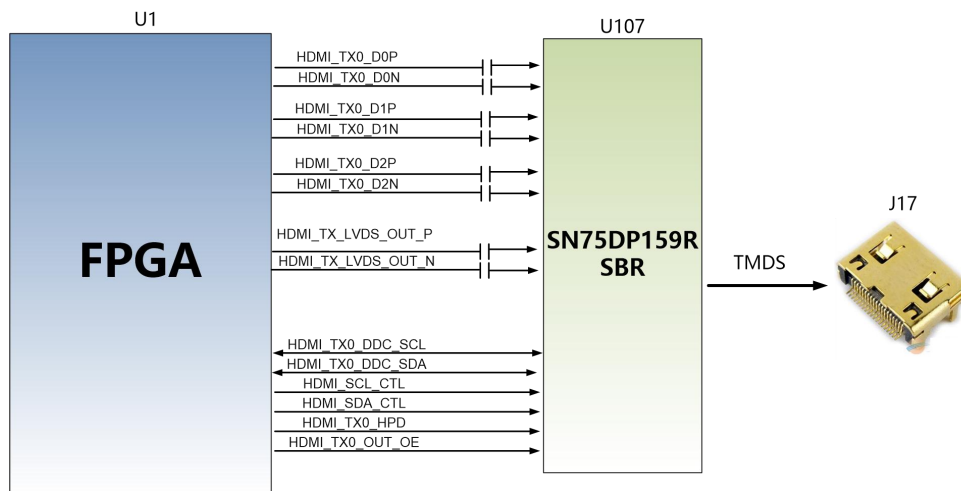
图 3-6-1 HDMI 输出接口设计示意图
