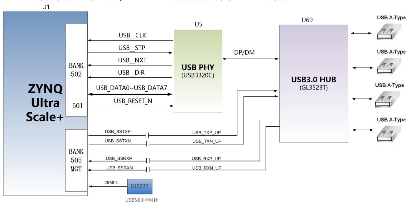
3-5-1 USB3.0 接口示意图
