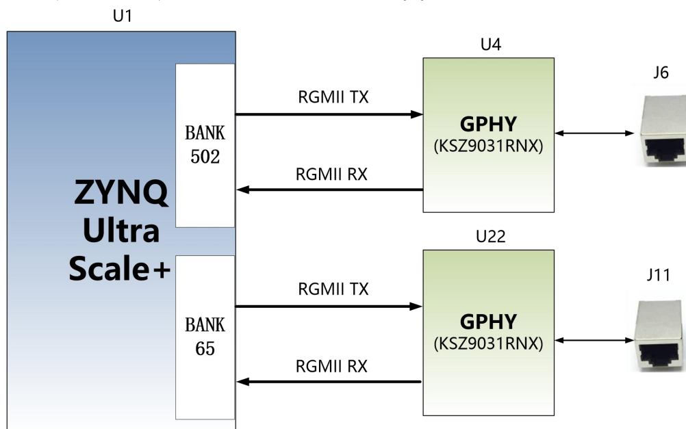
图 3-8-1 ZYNQ 与 GPHY 连接示意图
