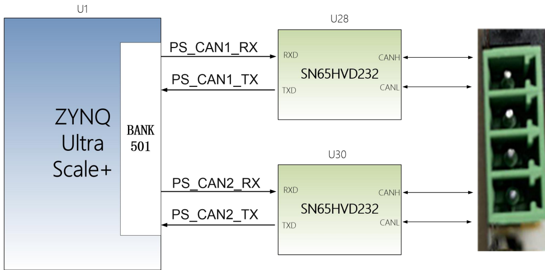
图 3-14-1 PS 端 CAN 收发芯片的连接示意图
