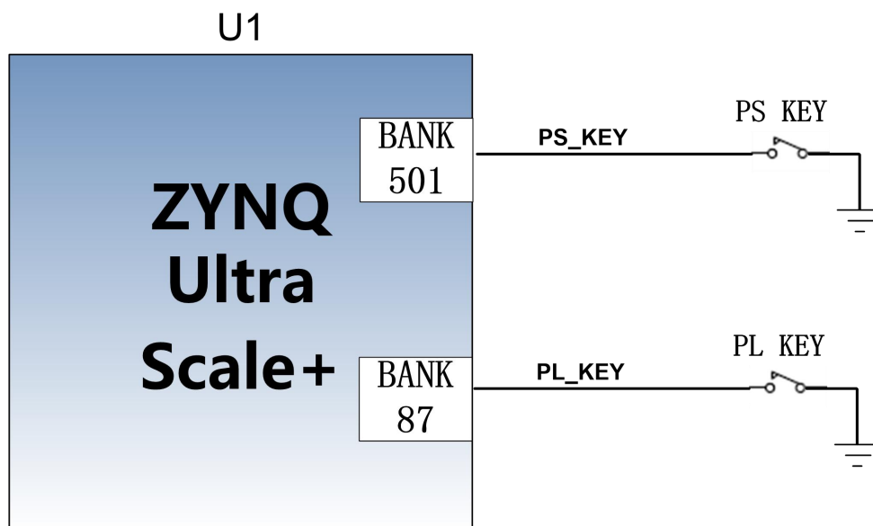
图 3-20-1 复位按键连接示意图
