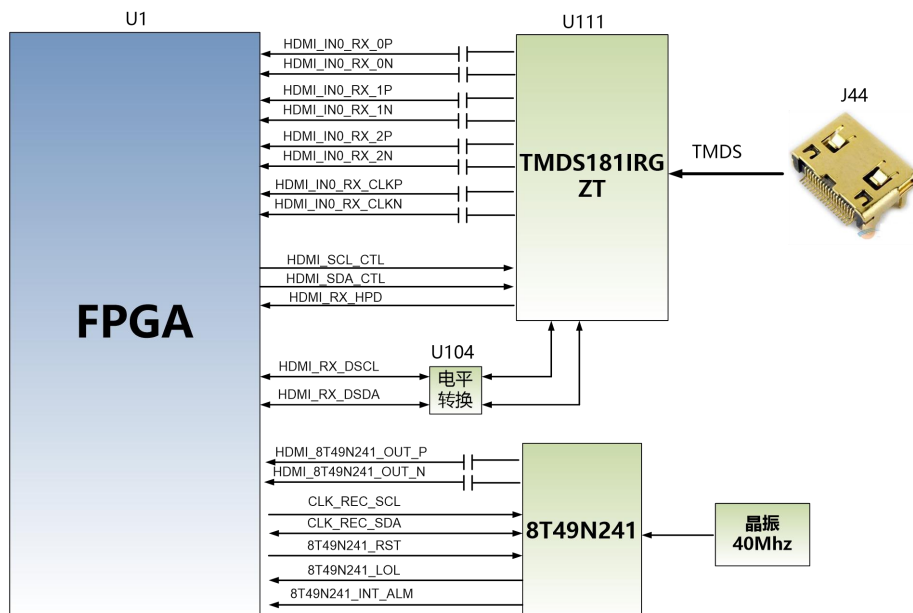
图 3-7-1 HDMI 输入接口设计示意图
