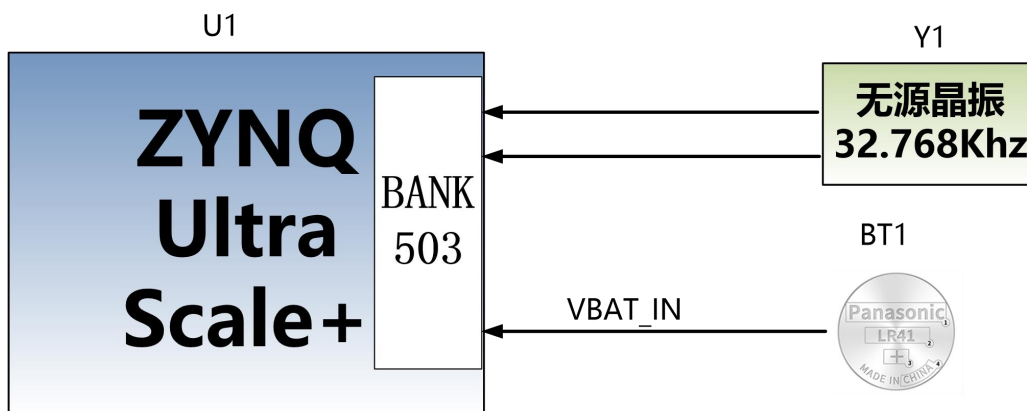
图 3-17-1 为 RTC 实时时钟原理图
