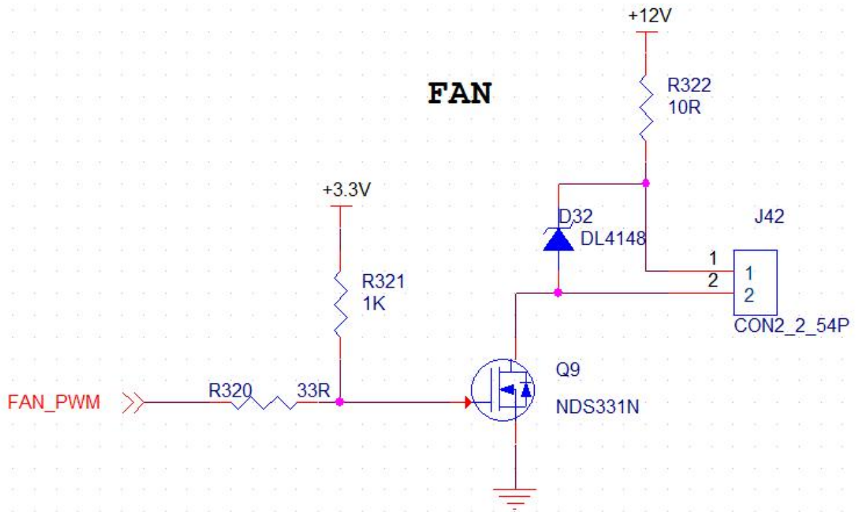
图 3-23-1 开发板风扇设计
