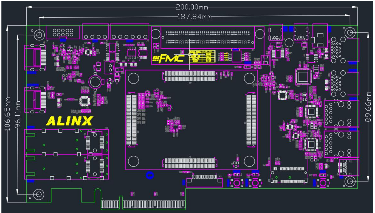
图 3-24-1 正面图 (Top View)
