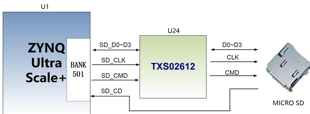
图 3-11-1 SD 卡连接示意图
