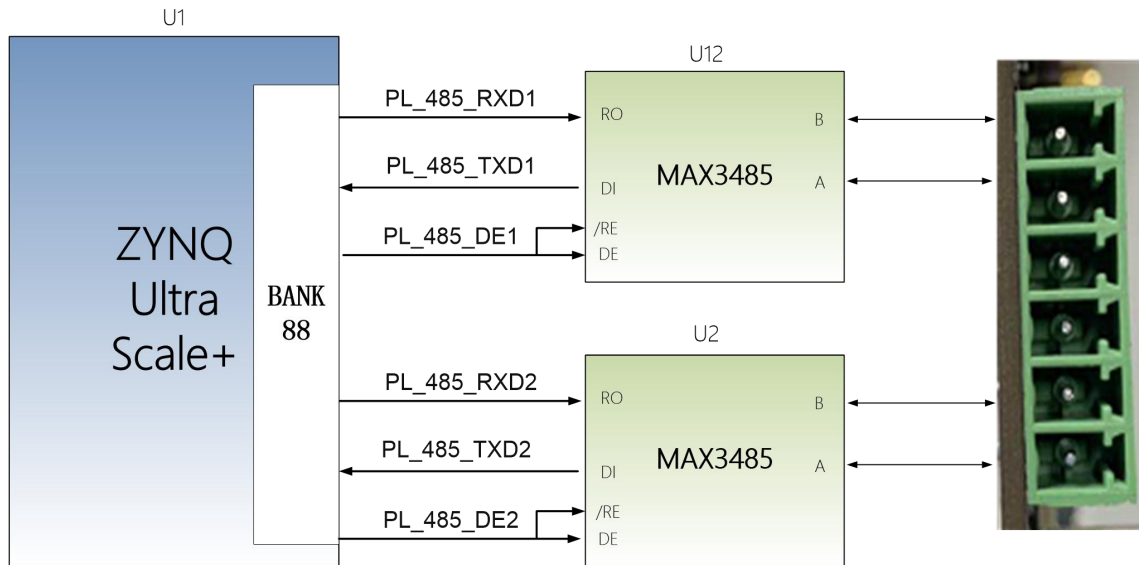
图 3-15-1 PL 端 485 通信的连接示意图
