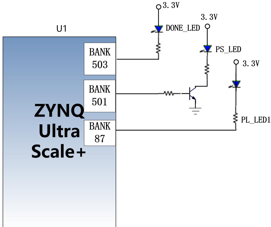
图 3-19-1 用户 LED 灯硬件连接示意图
