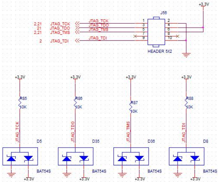
图3-16-1 原理图中JTAG接口部分
