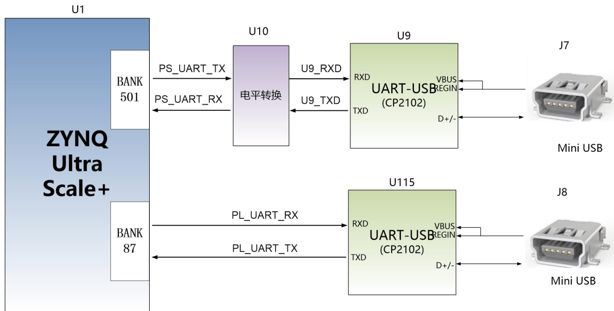
3-9-1 USB 转串口示意图
