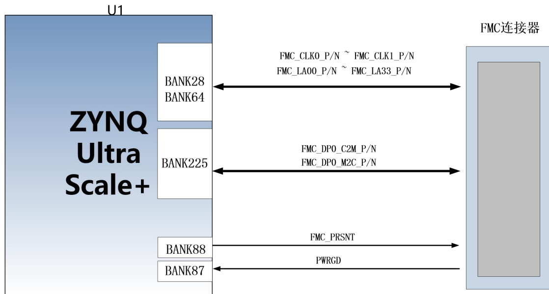
图 3-13-1 FMC 连接器连接示意图
