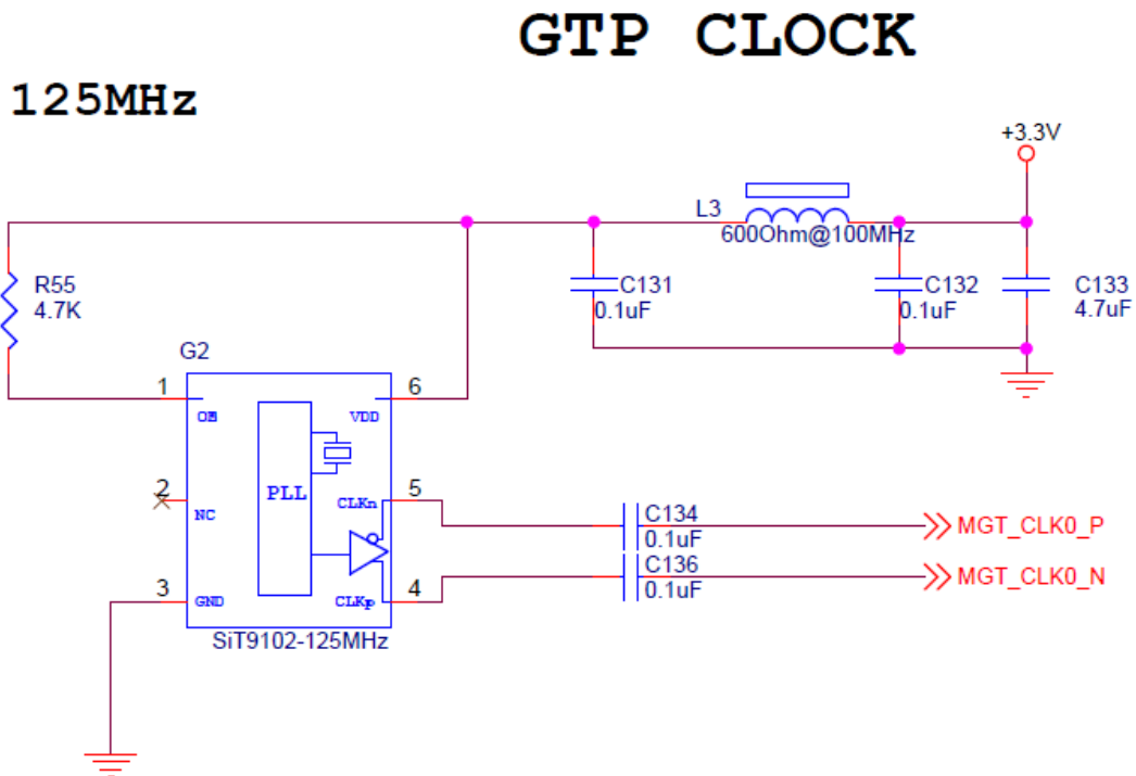
图 2-3-3 125Mhz 有源差分晶振
