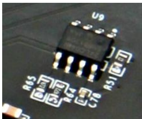
图 3-8-2 EEPROM 实物图
