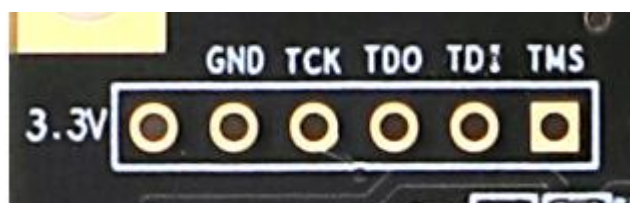
图 2-8-2 JTAG 接口实物图
